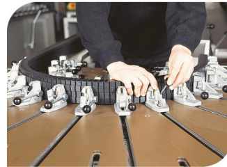
Ölçüsü Ayarlanmış Olan Şablonun Masaya Yerleştirilmesi
