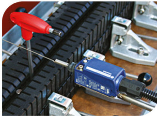
Bacaklı Bükümlerde Çekme Motorunu Durduran Switch
